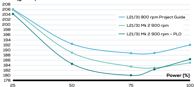
SFOC [g/kWh]
