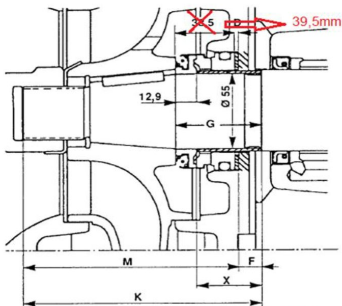
FIG.3 : AJUSTAGE DE L'ENTRETOISE ET DE LA CALE SPACER AND SHIM ADJUSTEMENT
